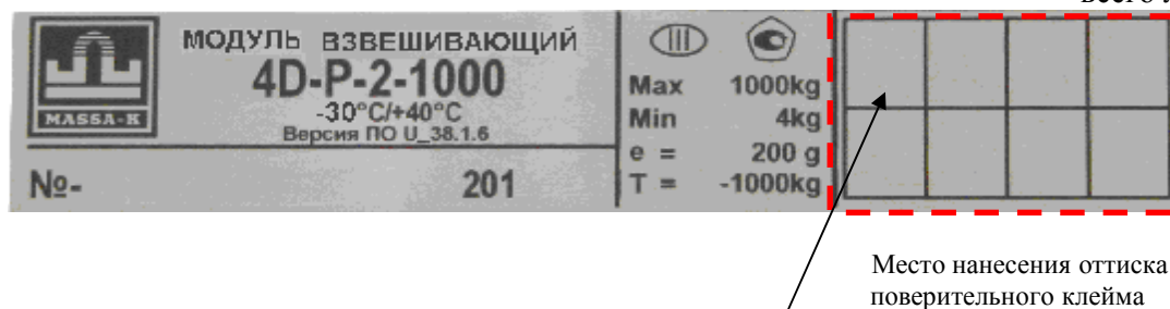
Рисунок 4 – Маркировка модуля взвешивающего и место нанесения оттиска поверительного клейма
